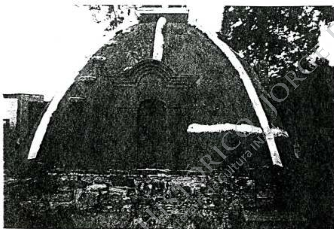
Vista general de la cúpula, dos lucernas tapiadas, recubrimiento con impermeabilizante asfáltico, presencia de grietas horizontales. Junio 2000
