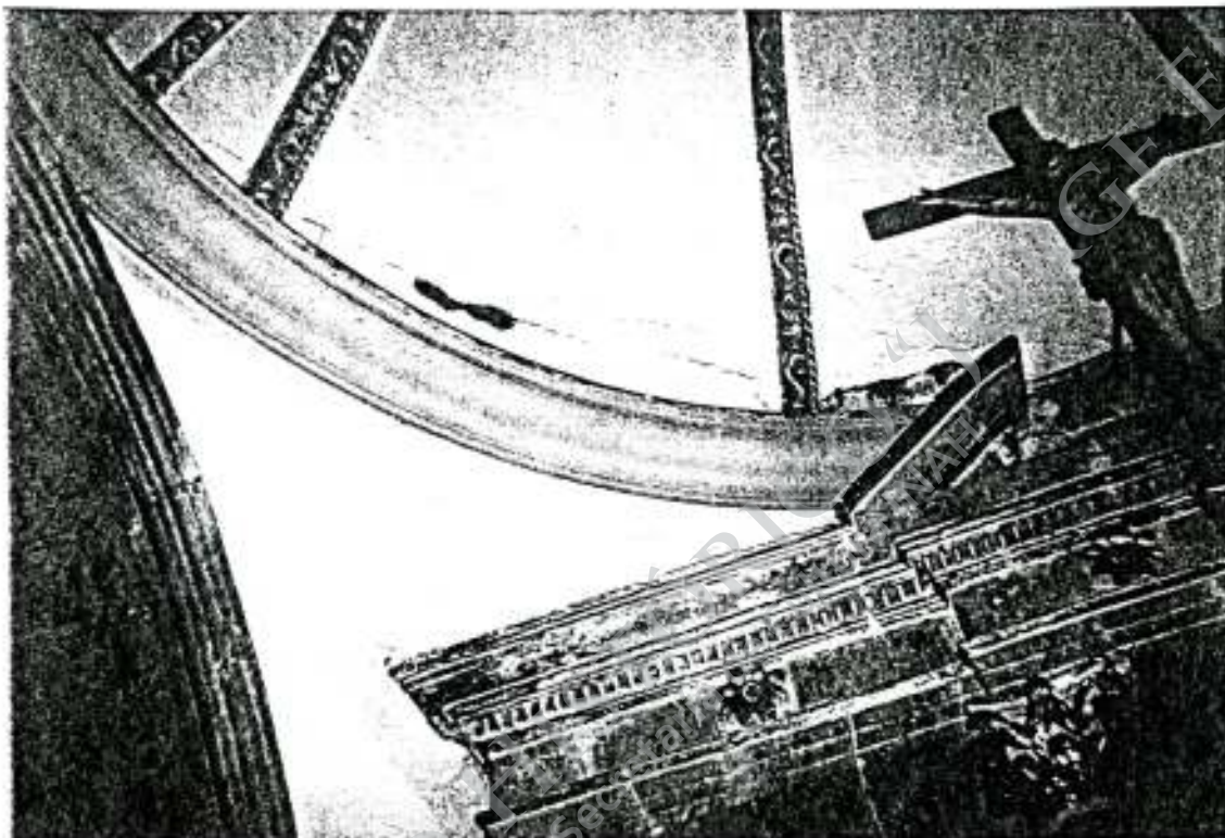
Vista superior del altar mayor, grieta continua paralela al arco de compresión, filtración de agua en pectinas y cúpula.
